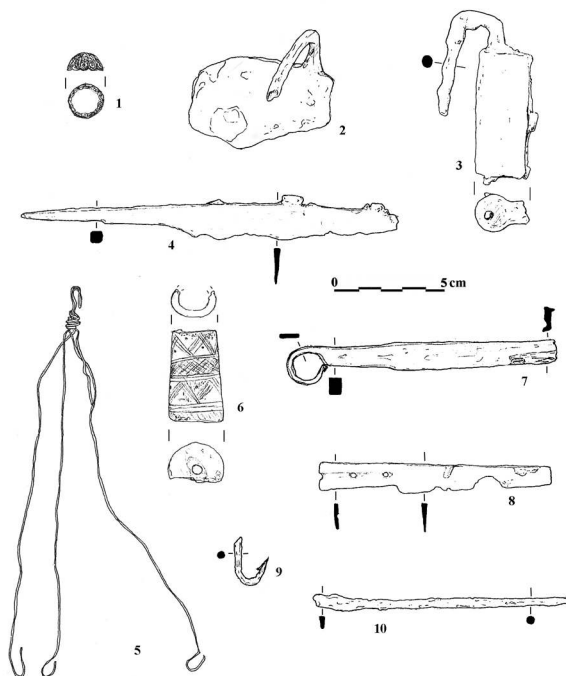
Сл. 8. Налази из цркве (1–3), сонде 5/14 (4) и конака (5–10)
